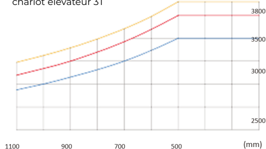
Courbe de charge chariot élévateur 3T
